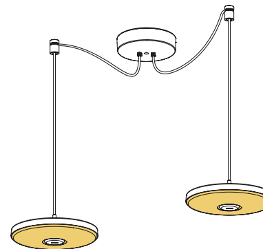
DISC PENDANT 100-230V DUO
